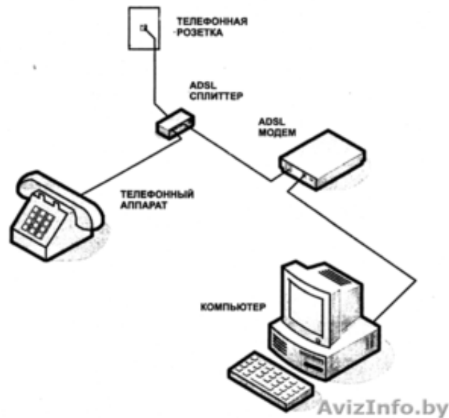
Схема подключения ADSL-модема
